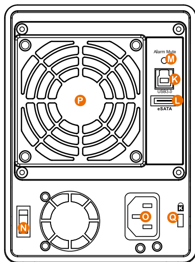
背面圖
